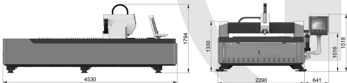
Figura 1. Vista lateral y frontal con medidas de FORZA RAPTOR 1500W sin equipos adicionales.
